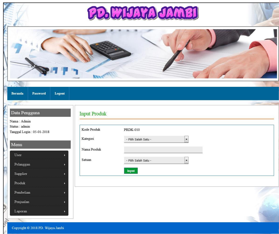
Gambar 5.16 Input Produk
