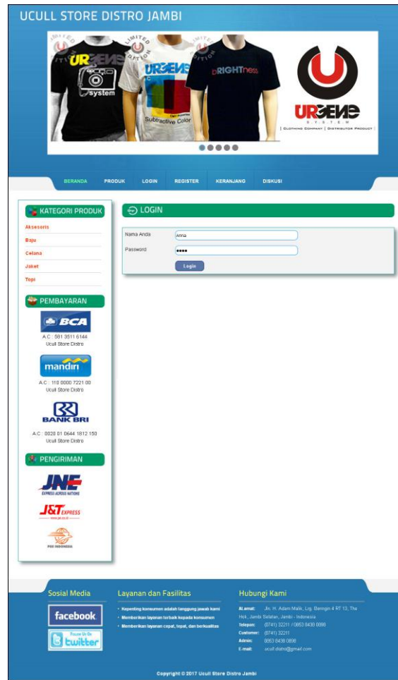
Gambar 5.6 Login
