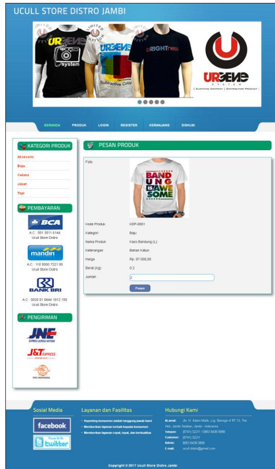
Gambar 5.9 Pesan Produk
