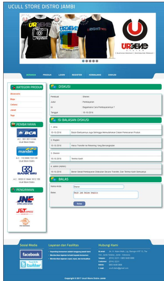
Gambar 5.8 Balas Diskusi
