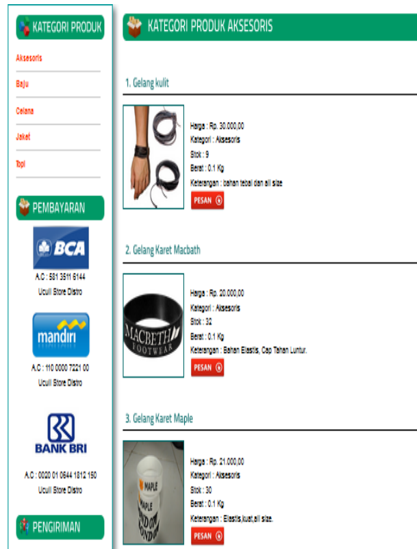
Gambar 5.16 Produk
