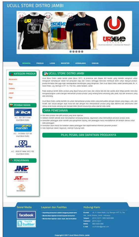
Gambar 5.15 Beranda Pengunjung
