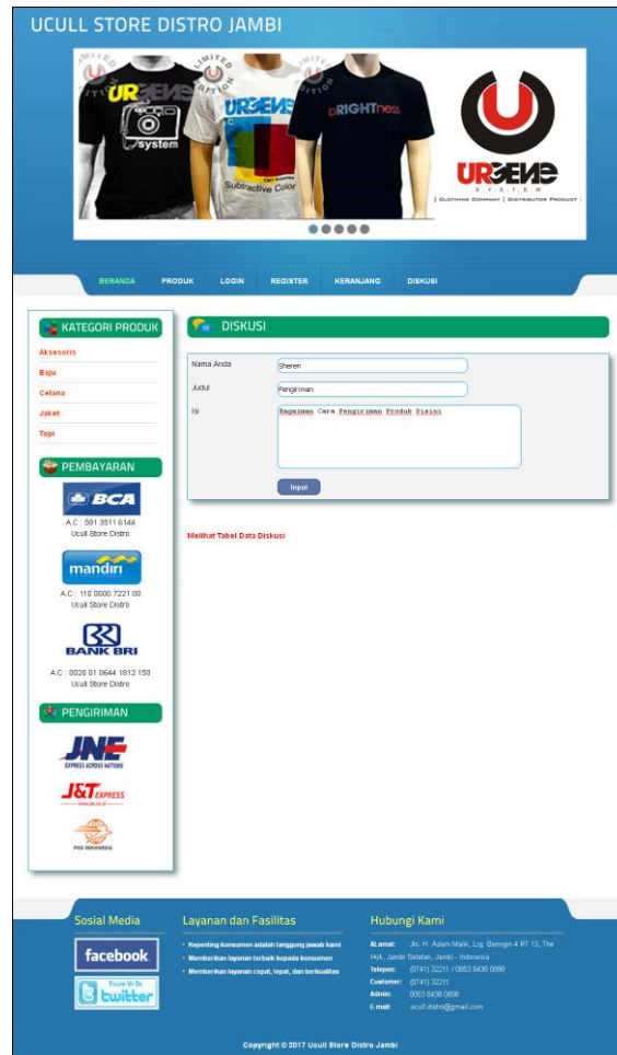
Gambar 5.7 Diskusi
