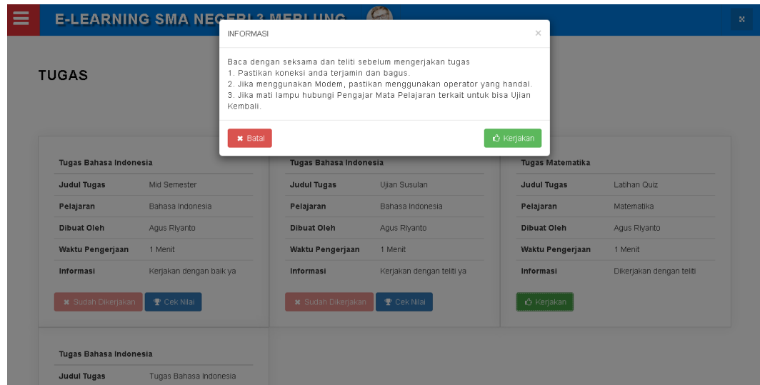
Gambar 5.8 Halaman Informasi
