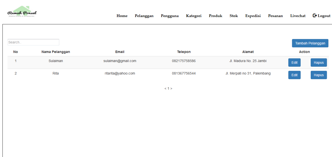
Gambar 5.7 Halaman Pelanggan
