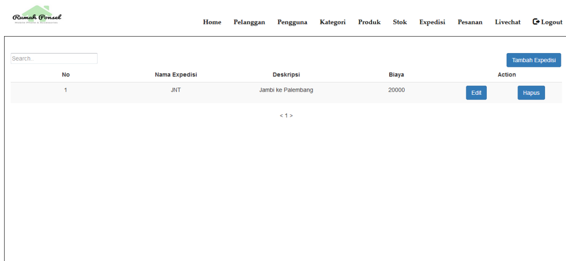
Gambar 5.12 Halaman Ekspedisi
