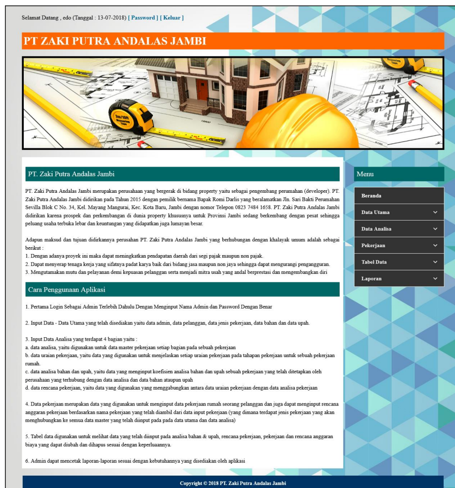
Gambar 5.13 Beranda
