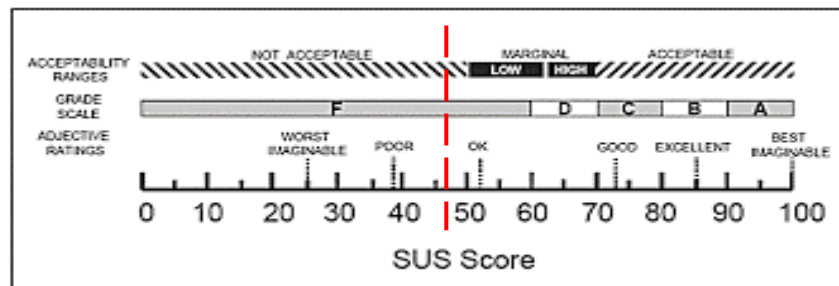
Gambar 5.18 Skor SUS
