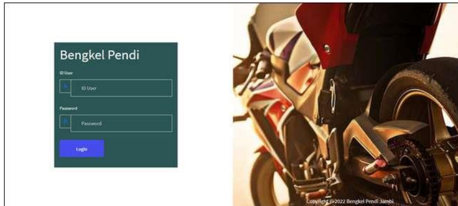
Gambar 5.9 Halaman Login
