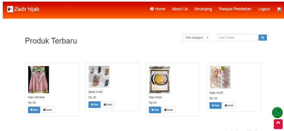
Gambar 5.3 Produk & Belanja
