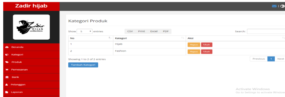
Gambar 5.10 Kategori Produk
