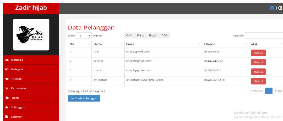
Gambar 5.11 Data Pelanggan
