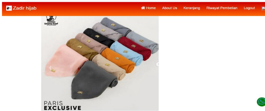
Gambar 5.1 Beranda Pengunjung
