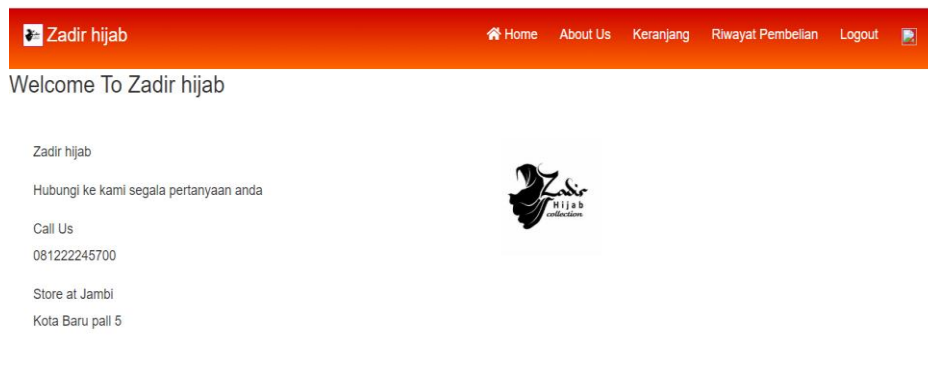
Gambar 5.4 Profil Toko
