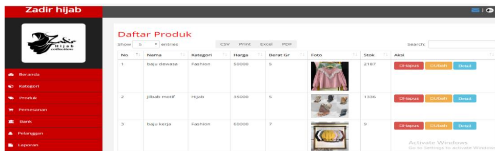
Gambar 5.9 Data Produk
