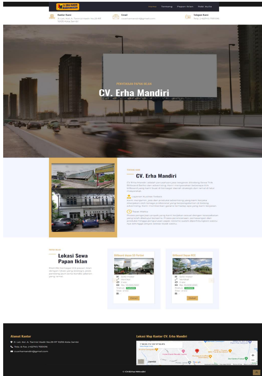
Gambar 5. 16 Halaman Utama
