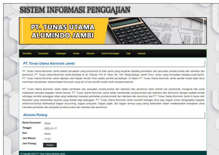
Gambar 5.1 Halaman Beranda
