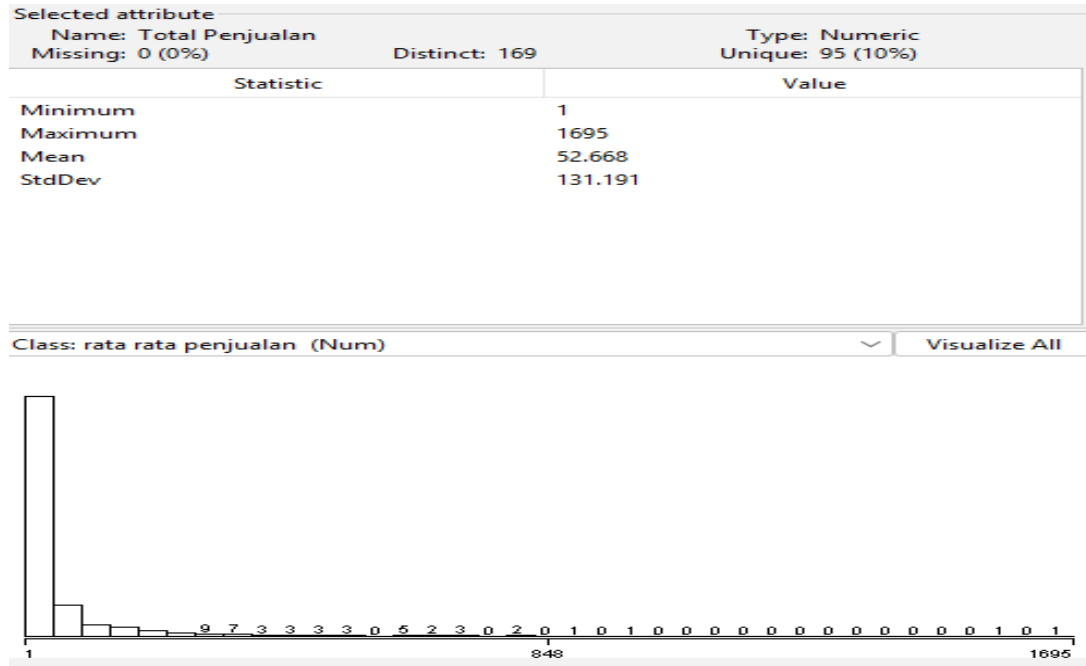
Gambar 5.4 Visualisasi Atribut Total Penjualan
