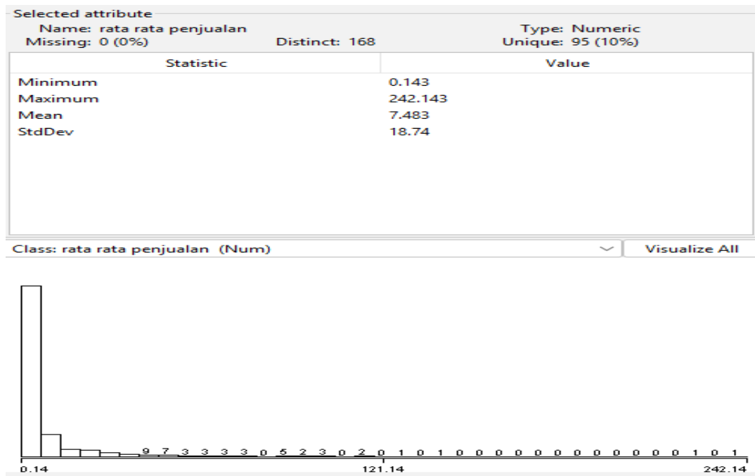
Gambar 5.5 Visualisasi Atribut Rata – rata Penjualan
