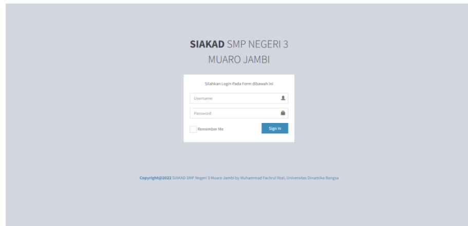
Gambar 5.1 Halaman Login
