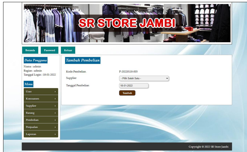
Gambar 5.8 Tambah Pembelian
