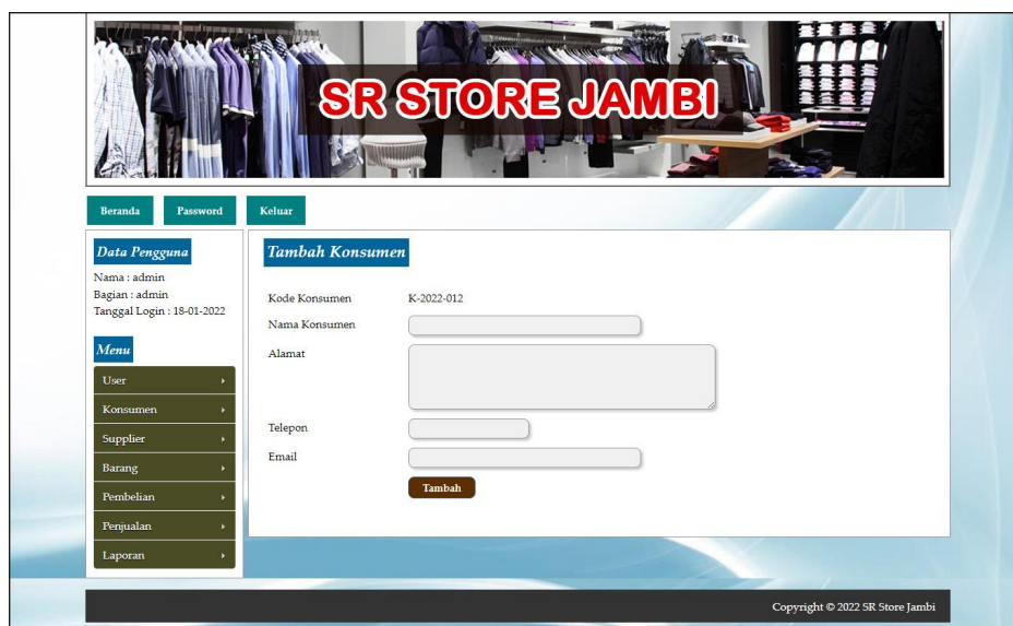
Gambar 5.4 Tambah Konsumen
