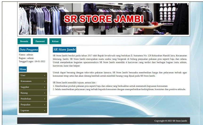
Gambar 5.2 Halaman Beranda
