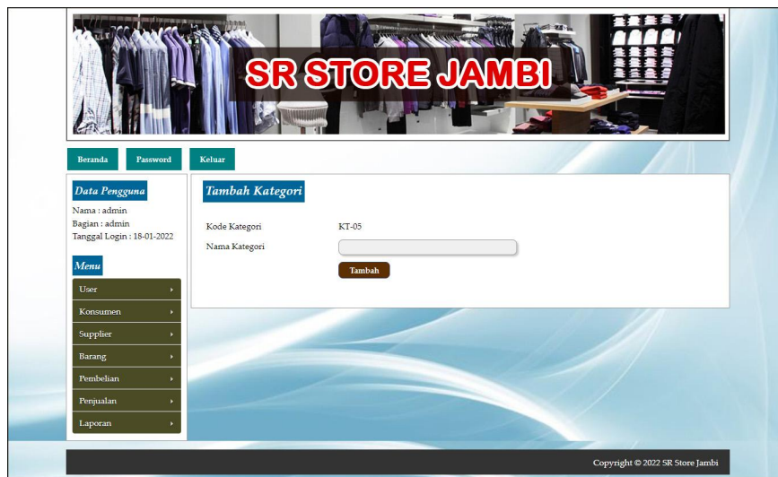
Gambar 5.6 Tambah Kategori
