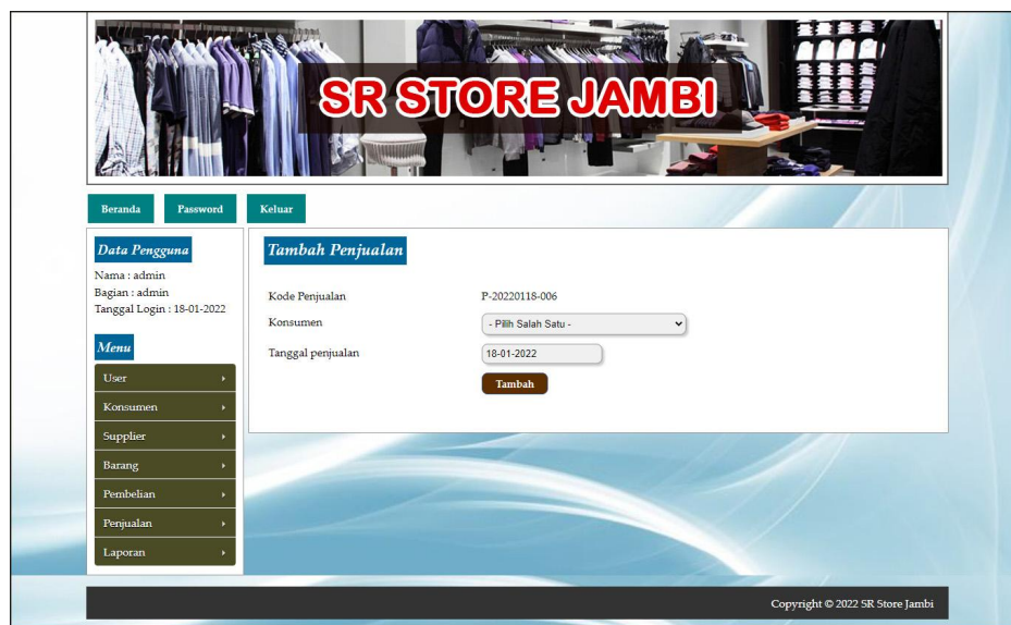
Gambar 5.10 Tambah Penjualan
