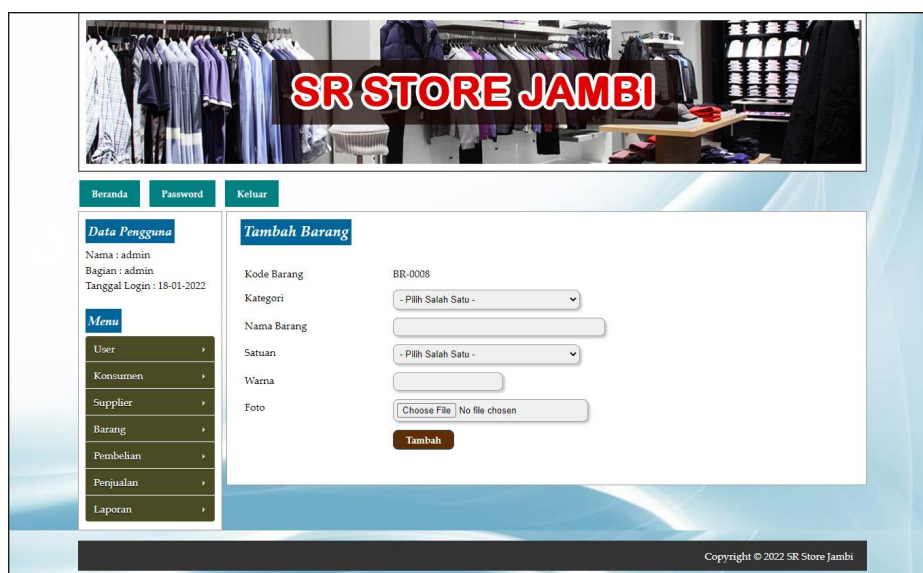
Gambar 5.7 Tambah Barang
