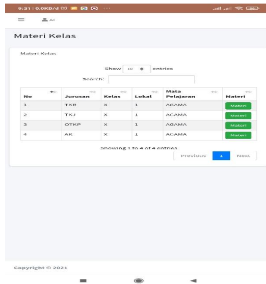
Gambar 5.11 Tampilan Halaman Mengelola Materi
