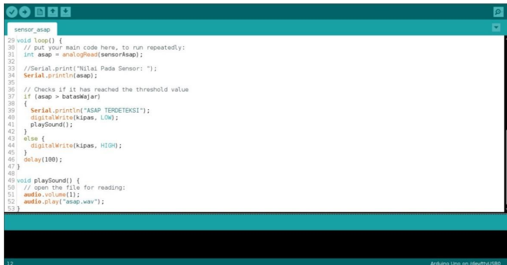
Gambar 5.4 Penggalan Sketch Program Logika If
