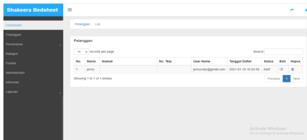
Gambar 5.13 Data Pelanggan
