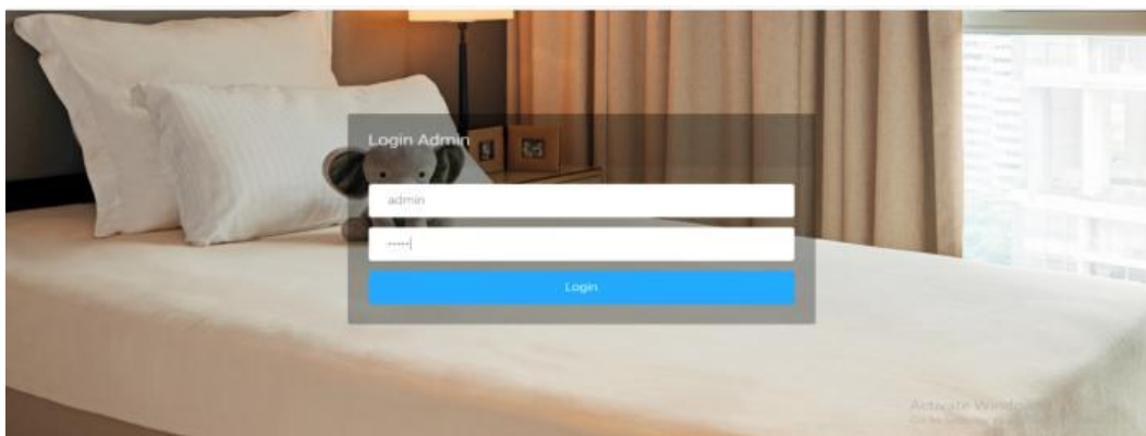
Gambar 5.1 Halaman Login
