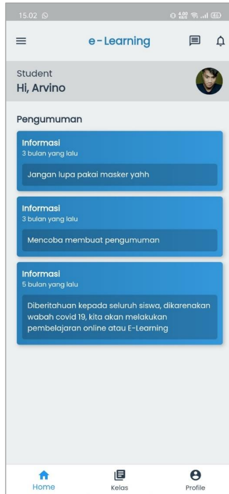
Gambar 5.20 Halaman Utama
