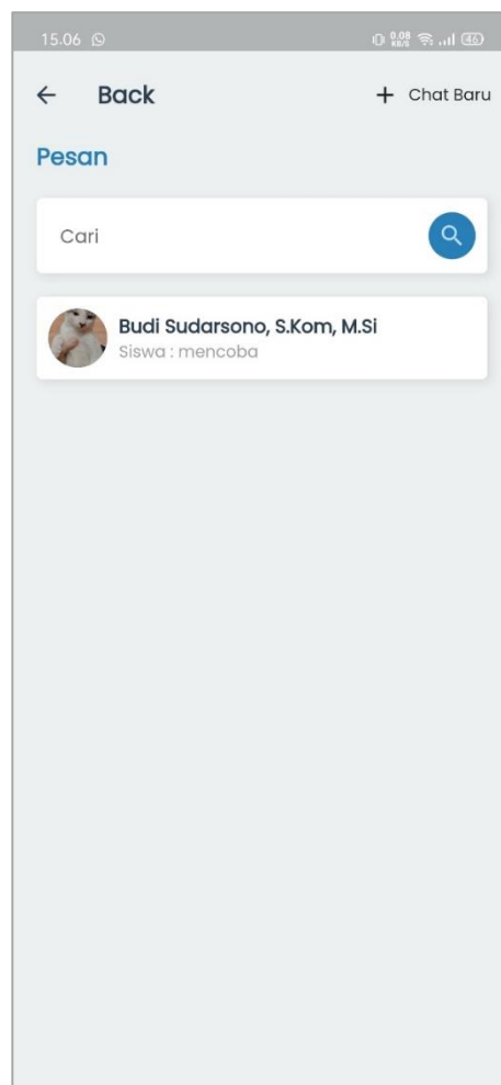
Gambar 5.30 Halaman Pesan
