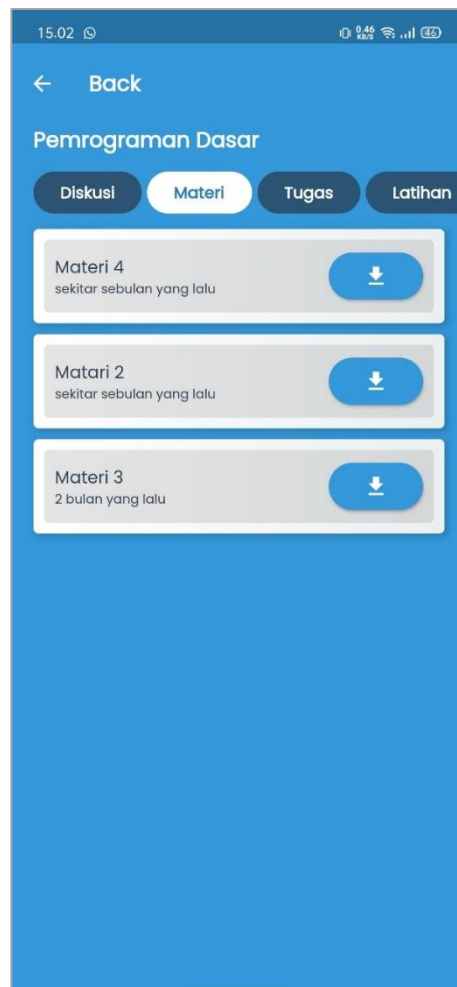
Gambar 5.25 Halaman Materi
