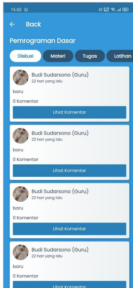
Gambar 5.23 Halaman Diskusi
