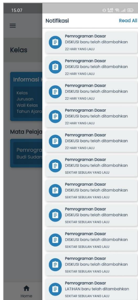
Gambar 5.32 Halaman Notifikasi
