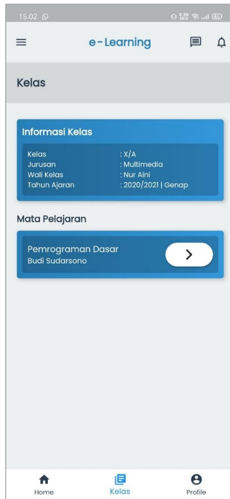
Gambar 5.21 Halaman Kelas
