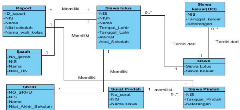
Gambar 5.3 Class diagram pelepasan siswa
