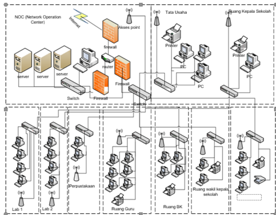
Gambar 5.9 Topologi Jaringan
