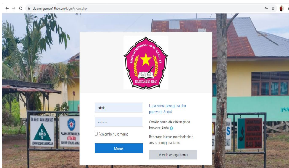
Gambar 5.1 Halaman Login
