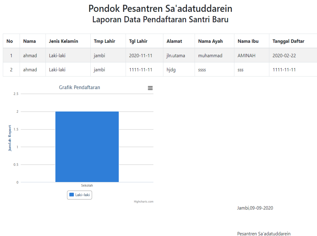
Gambar 5.17 Tampilan Output Laporan Data Pendaftaran Siswa Baru
