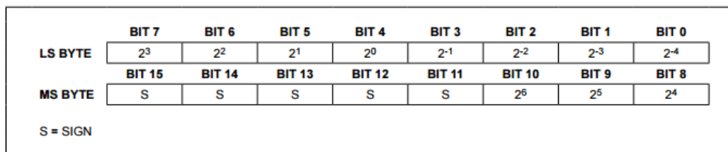
Gambar 5.1 Format Register Suhu pada DS18b20 (Sumber : www.maximintegrated.com )
