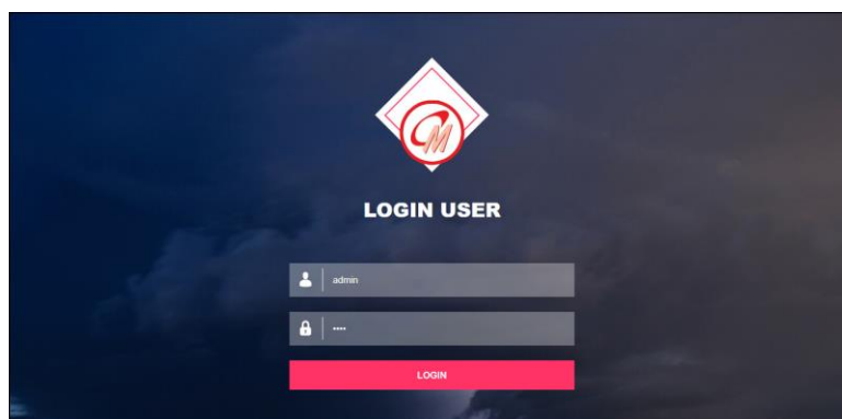
Gambar 5.12 Login
