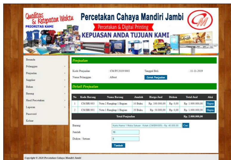
Gambar 5.15 Detail Penjualan
