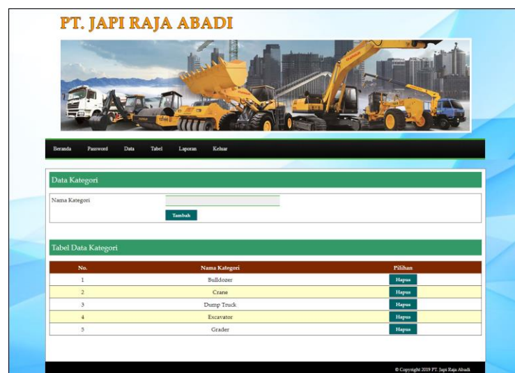
Gambar 5.9 Data Kategori
