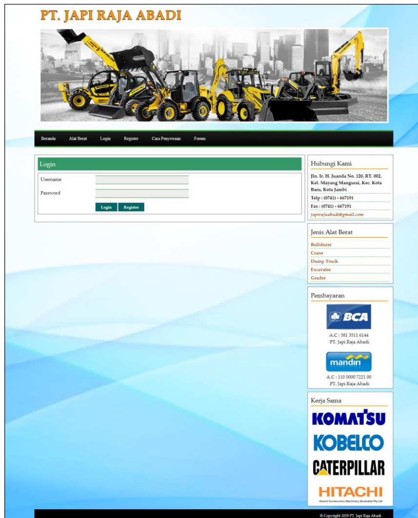
Gambar 5.5 Login
