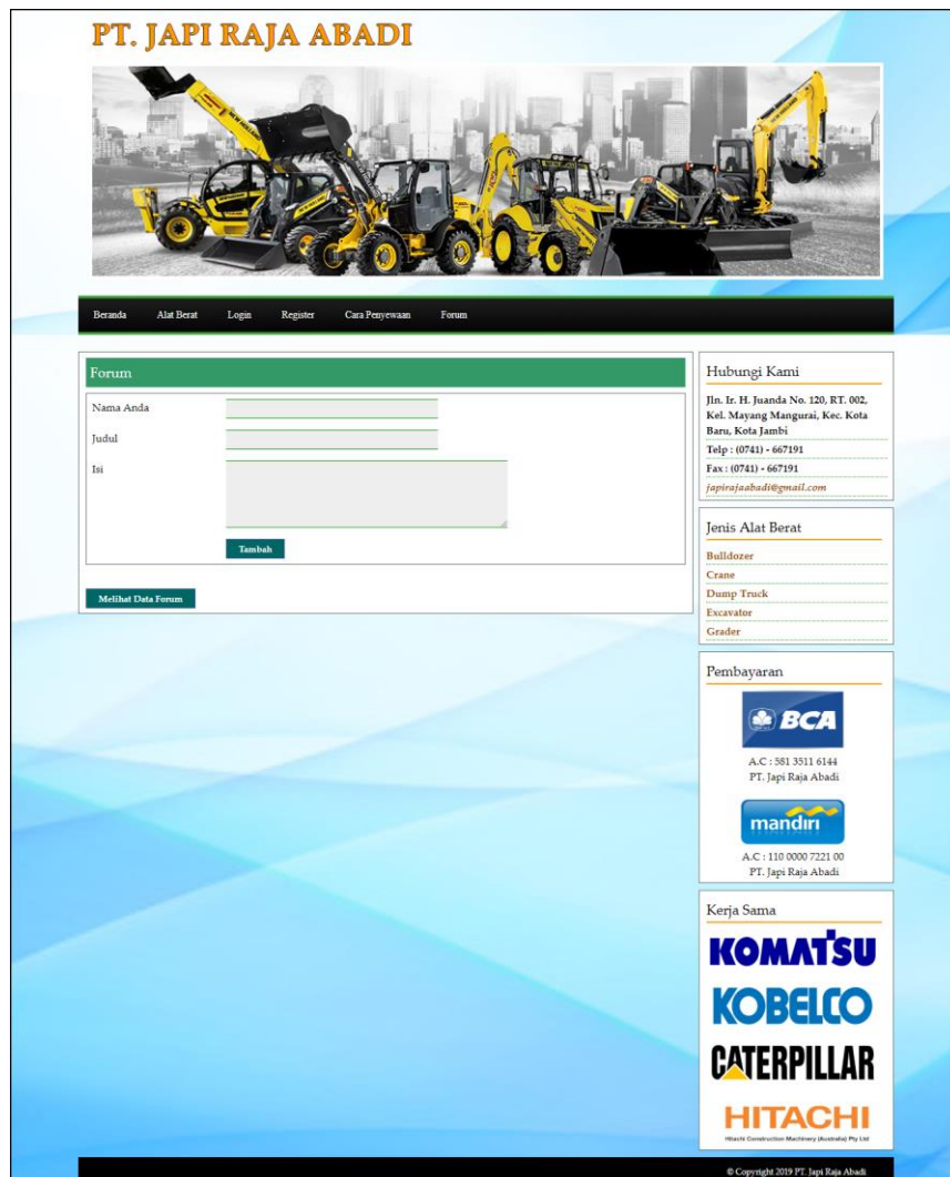
Gambar 5.3 Mengisi Forum
